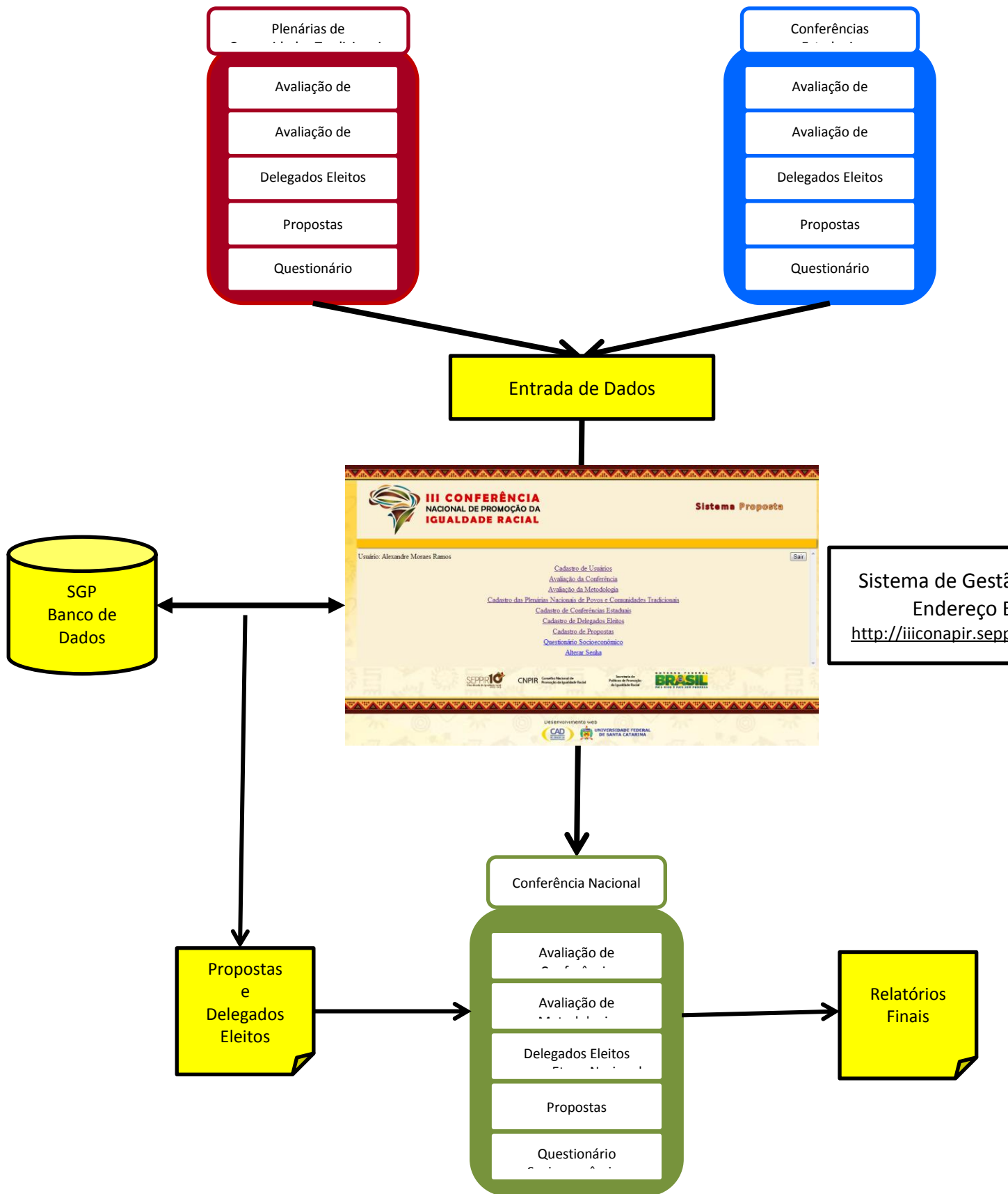
Figura 01 – Visão Geral do Sistema de Gestão de Propostas (SGP)
